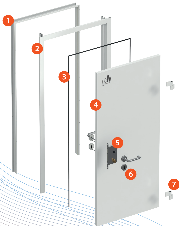
Рисунок 1. Технологическая дверь
